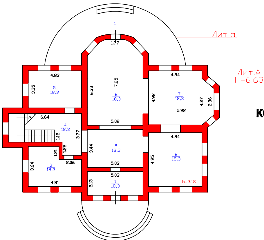
План I этажа
